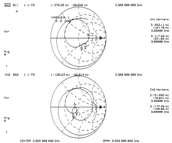
Zin, Zout
