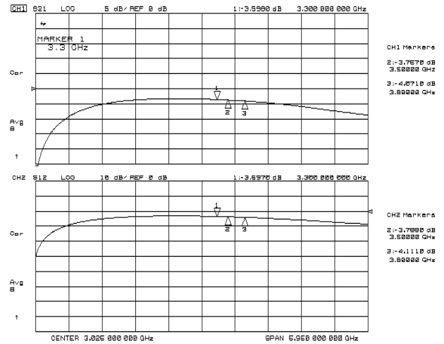
S21, S12
