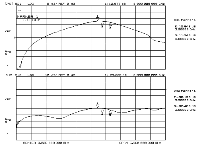
S21, S12
