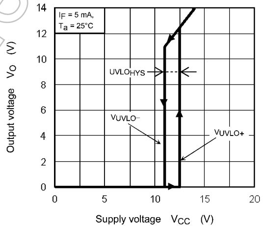
Fig. 12.2.12 V_O(V_{UVLO}) - V_{CC}
